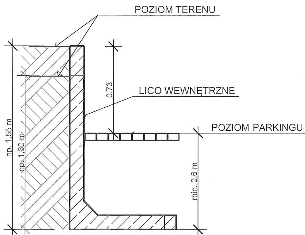
SCHEMAT MONTAŻU PREFABRYKATU
